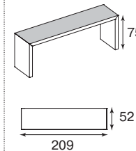
Каркас греденции 1511715015 2232
